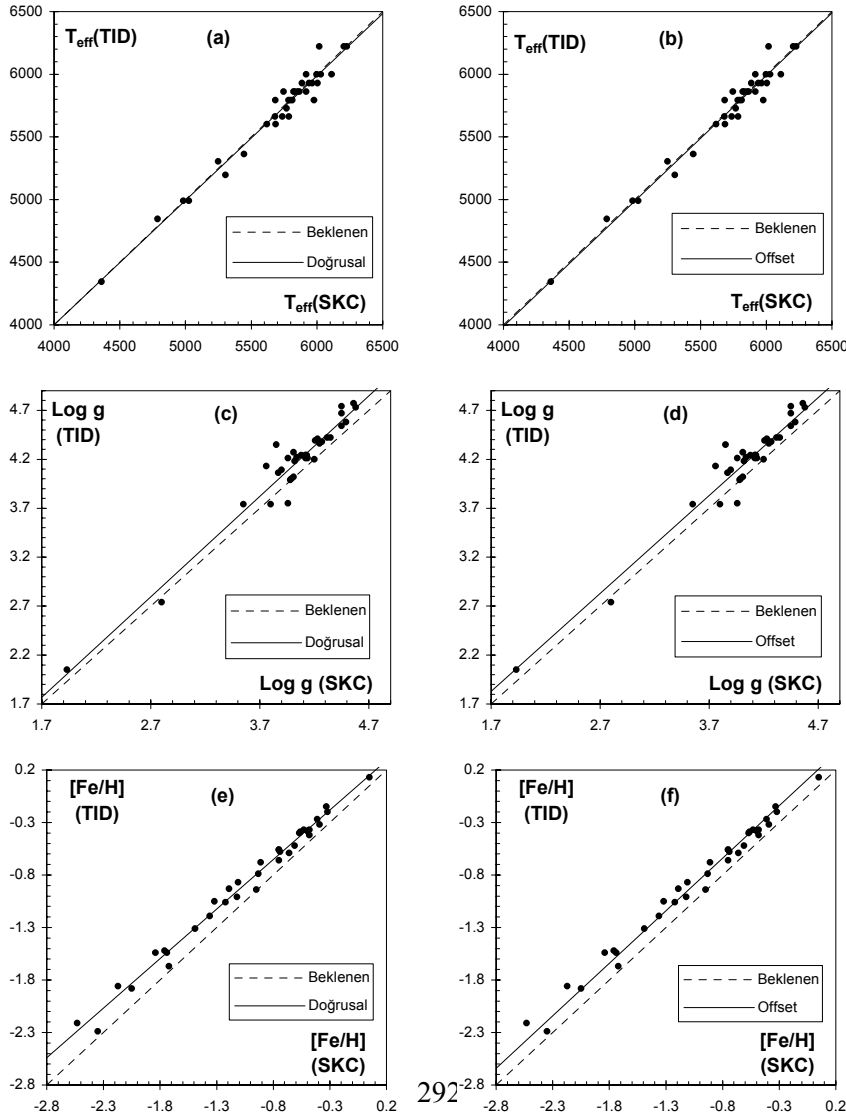
Şekil.1 Thevenin ve Idiart, 1999 (TID) atmosferik parametrelerinin SKC sistemine kalibrasyonu
