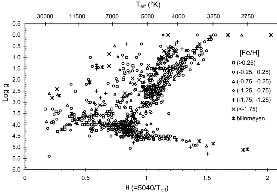
Şekil.2 Kütüphane yıldızları için sıcaklık-çekim ivmesi diyagramı
