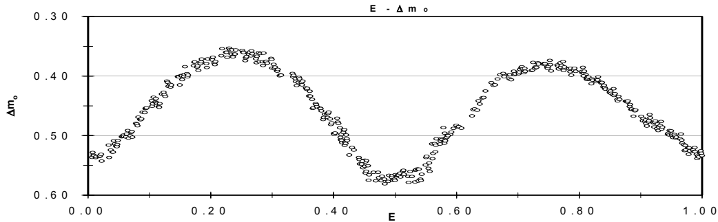
Şekil – 2 : OU Ser Yıldızının Işık Eğrisi (Değişen - Mukayese)
