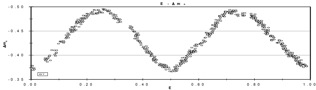
Şekil – 1 : V2150 Cyg Yıldızının Işık Eğrisi (Değişen - Mukayese)
