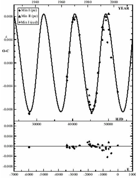
Şekil 2. AR Aur için oluşturulan en olası kuramsal O-C eğrisi ve gözlemler ile uyumu.
