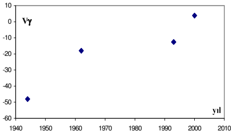
Şekil 6. UV Leo'nun yayınlanmış gamma hızlarının zaman bağılı değişimi.
