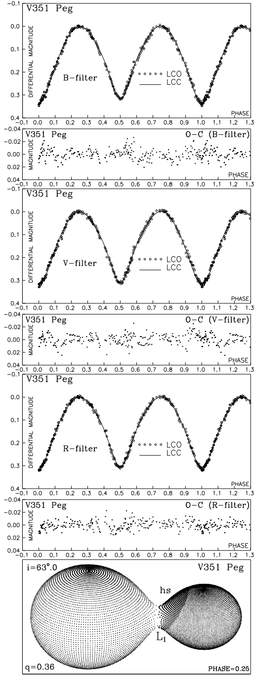
Şekil 2. V351 Peg'in teorik ile gözlemsel ışık eğrileri ve farkları, sistemin 0.25 evresindeki geometrik model
