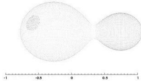
Şekil 2. Sistemin BVR bandlarındaki ışık eğrisine ilk yaklaşım olarak yapılan karşıtırmalar ve geometrik modeli.
