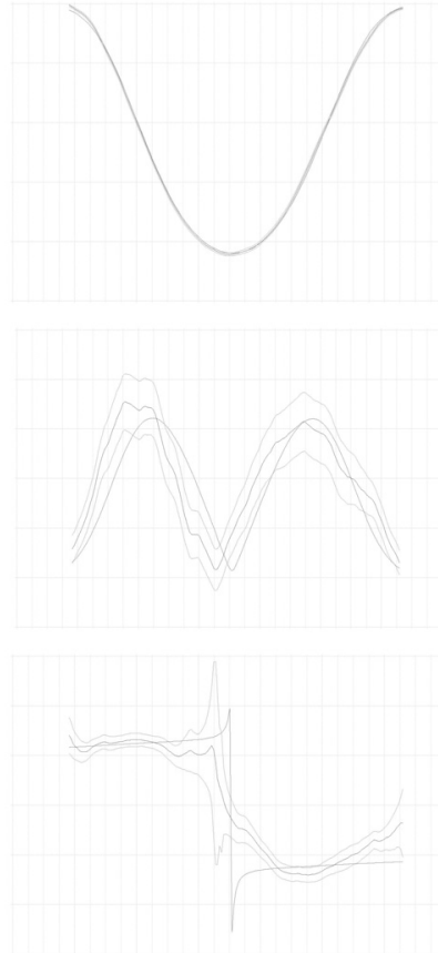
Şekil 2. EE Cam yıldızının çizgi profiline Fourier parametre yaklaşımının uyarlanması görülmektedir. En üst şekil sıfır-nokta
